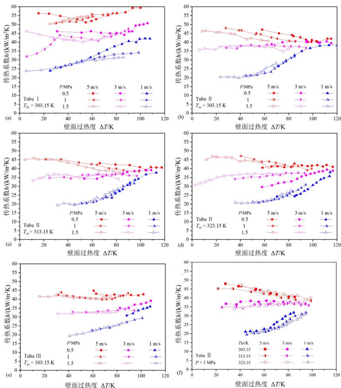
图4 微纳表面过冷流动沸腾传热系数随壁面过热度的变化
