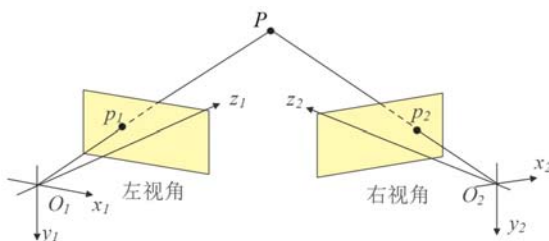
图 2 3D-DIC 成像模型 Fig. 2 3D-DIC imaging model
