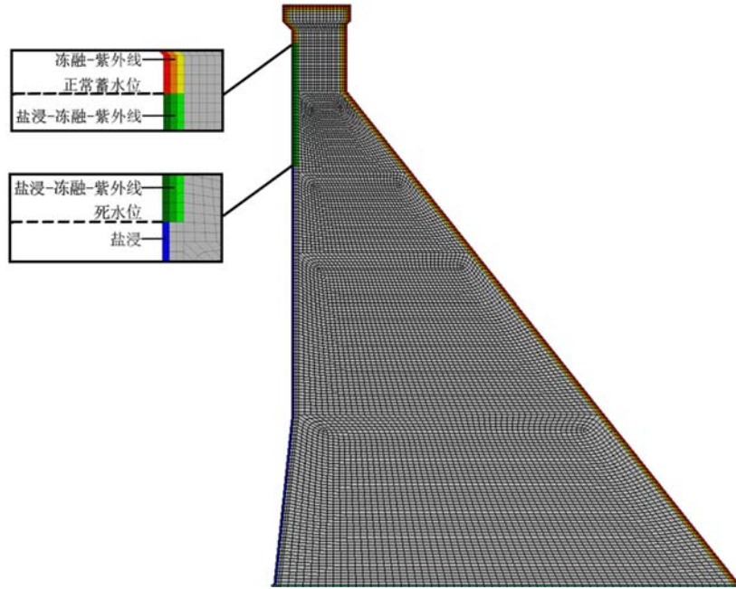
图 3 重力坝有限元模型
