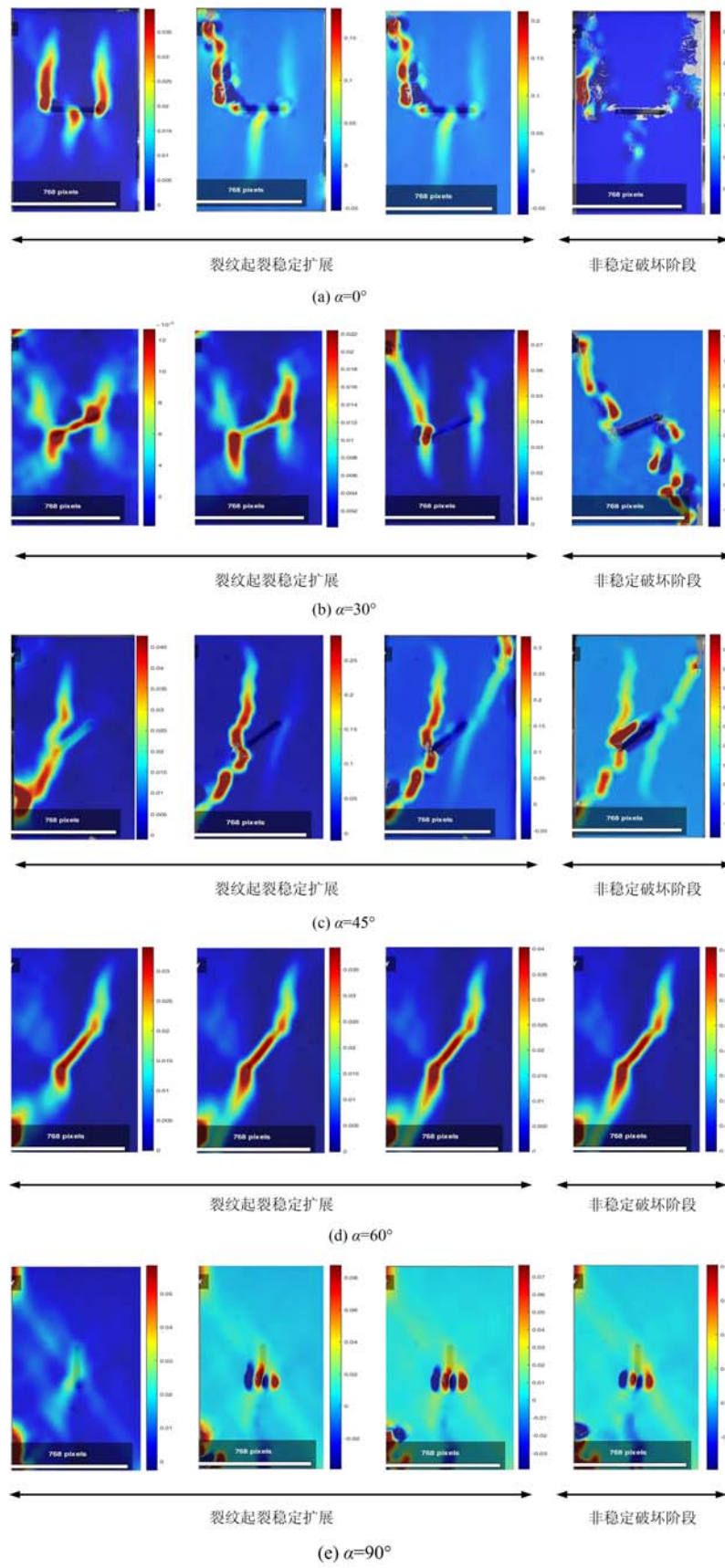
图 8 不同倾角裂隙岩石应变演化云图
